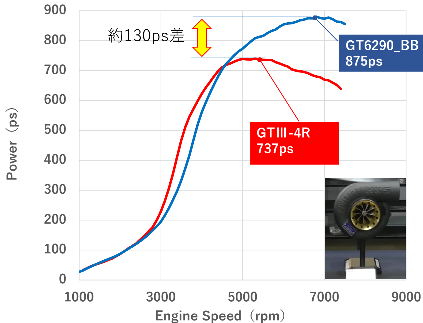
2J 3.4L × GT6290_BB 出力特性
