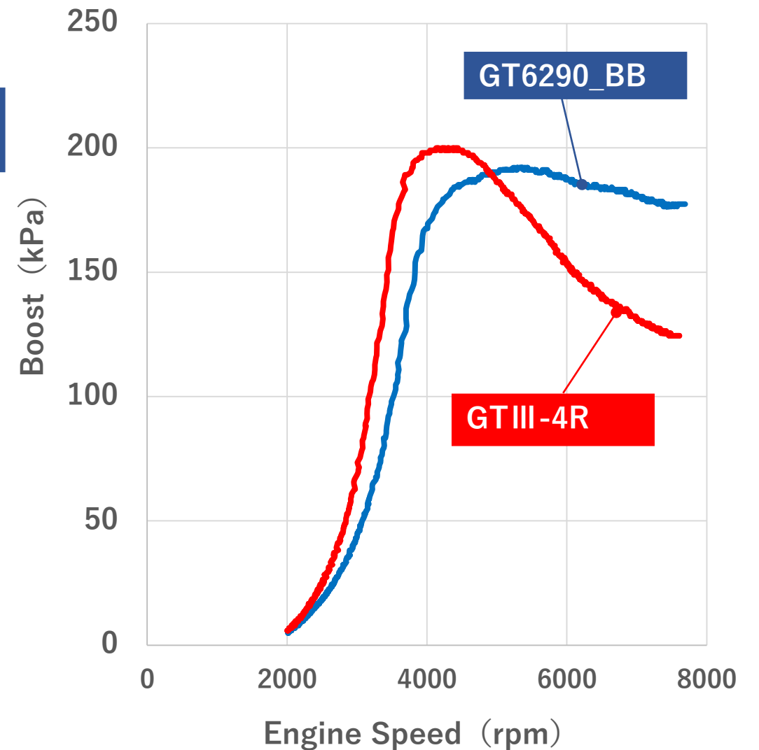
EVC150kPa (補正無し)設定時の過給圧特性
